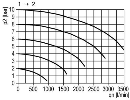
1. Durchflussdiagramm
