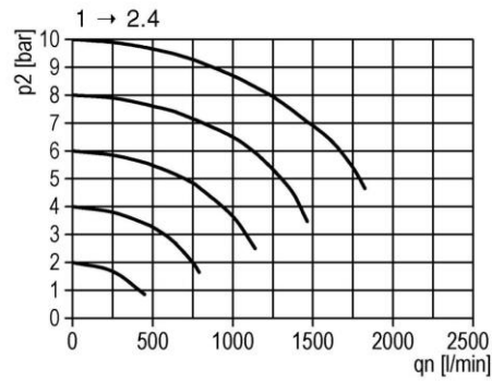
2. Durchflussdiagramm
